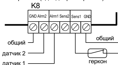
Пример 1. Подключение датчиков и герконов (одновверный режим)
