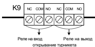
Пример 5. Подключение турникета (турникетный режим)
